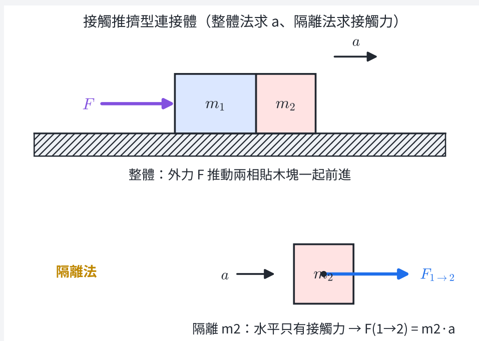
圖 4-6：接觸推擠型連接體。上排為整體情境：外力 F 推後塊 m_1 ， m_1 再推前塊 m_2 ，兩塊以同一加速度 a 前進。下排為前塊 m_2 的隔離自由體圖：水平方向只有 m_1 對它的接觸力 F_{1 \rightarrow 2} ，故
